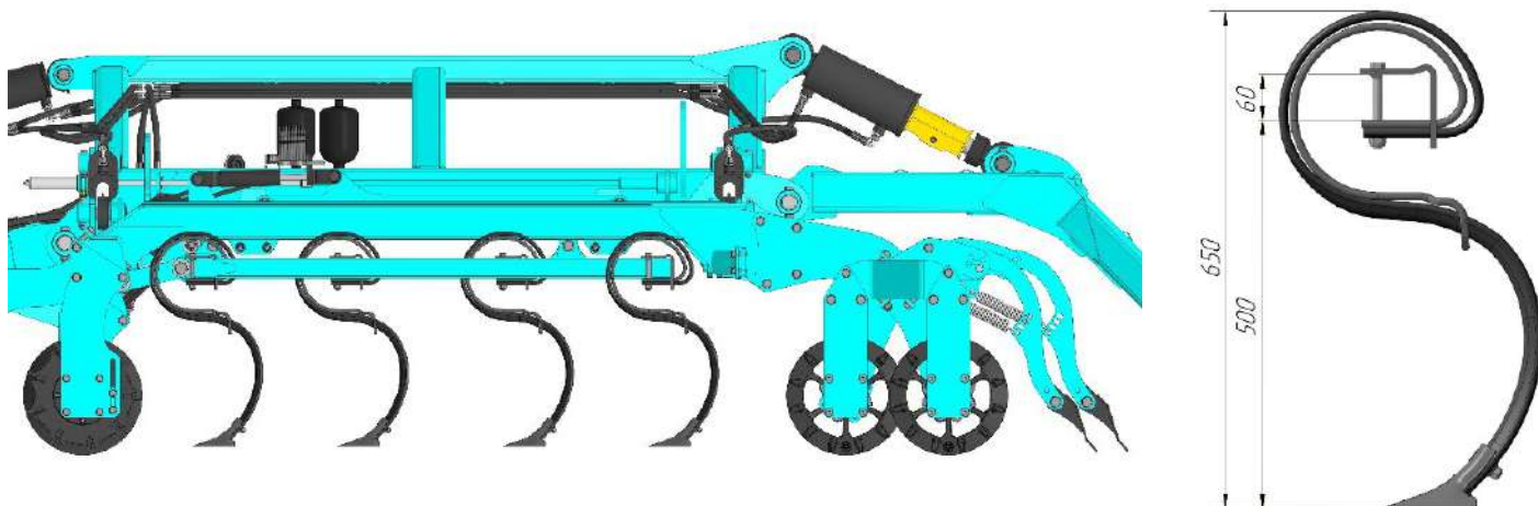
Рис. Четырехрядная секция
