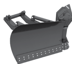
ОТВАЛ С ИЗМЕНЯЕМОЙ ГЕОМЕТРИЕЙ КРЫЛА (для УДМ, БКУ и ДМ15)
