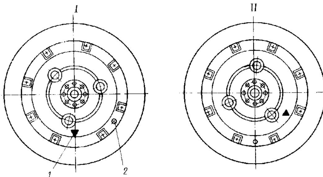
Рис. 82. Конечная передача
