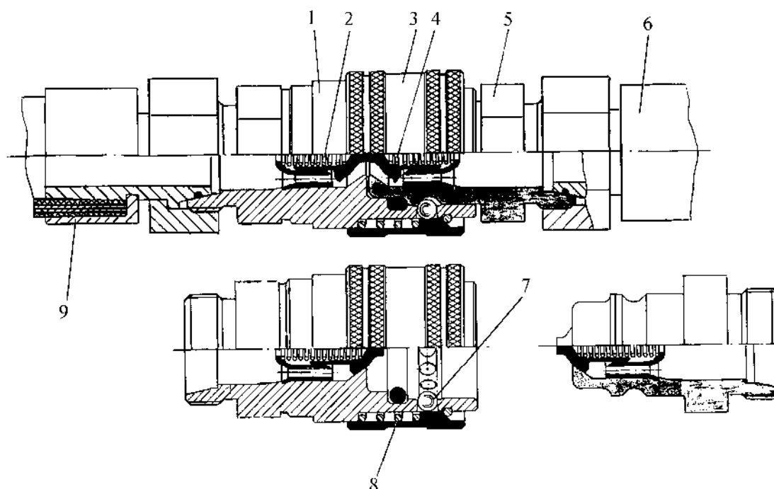
Рис. 71. Схема работы быстросоединяемых разрывных устройств
