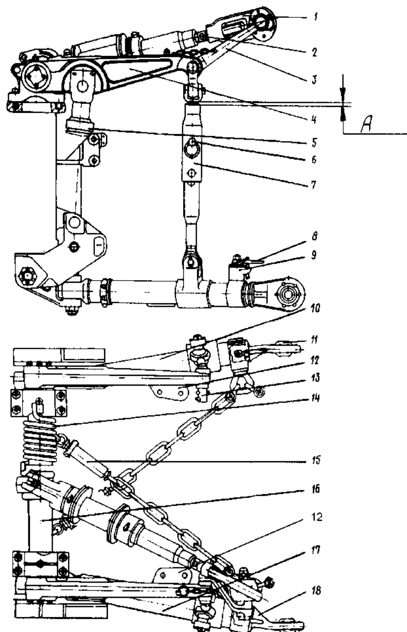
Рис. 72. Навесное устройство
