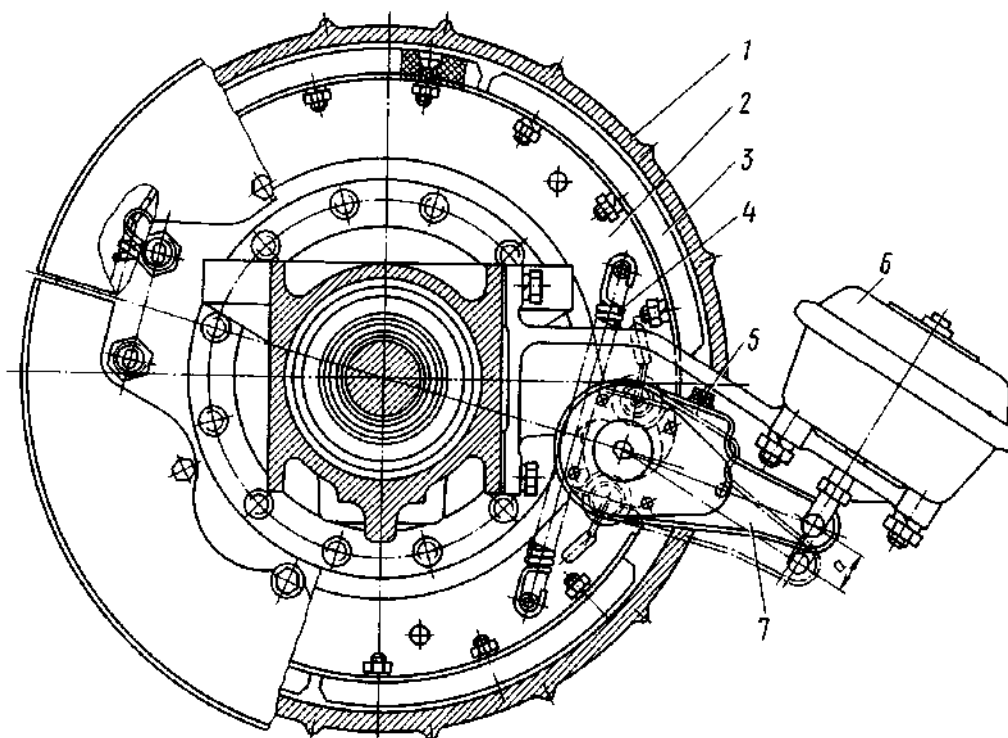
Рис. 83. Рабочий тормоз
