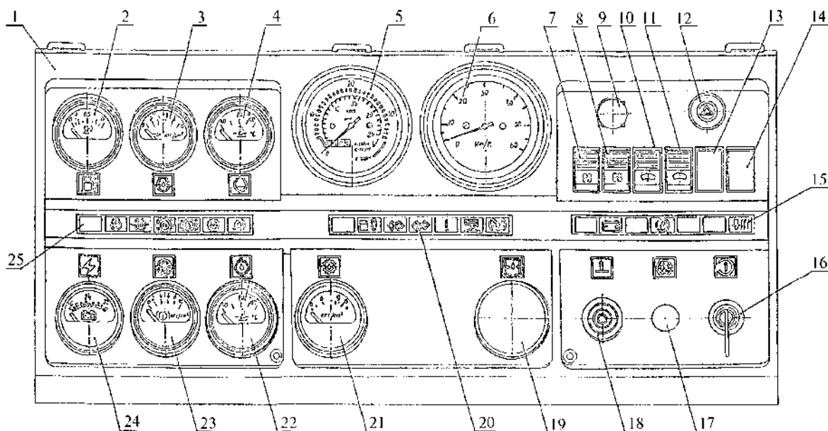
Рис. 2. Щиток приборов
