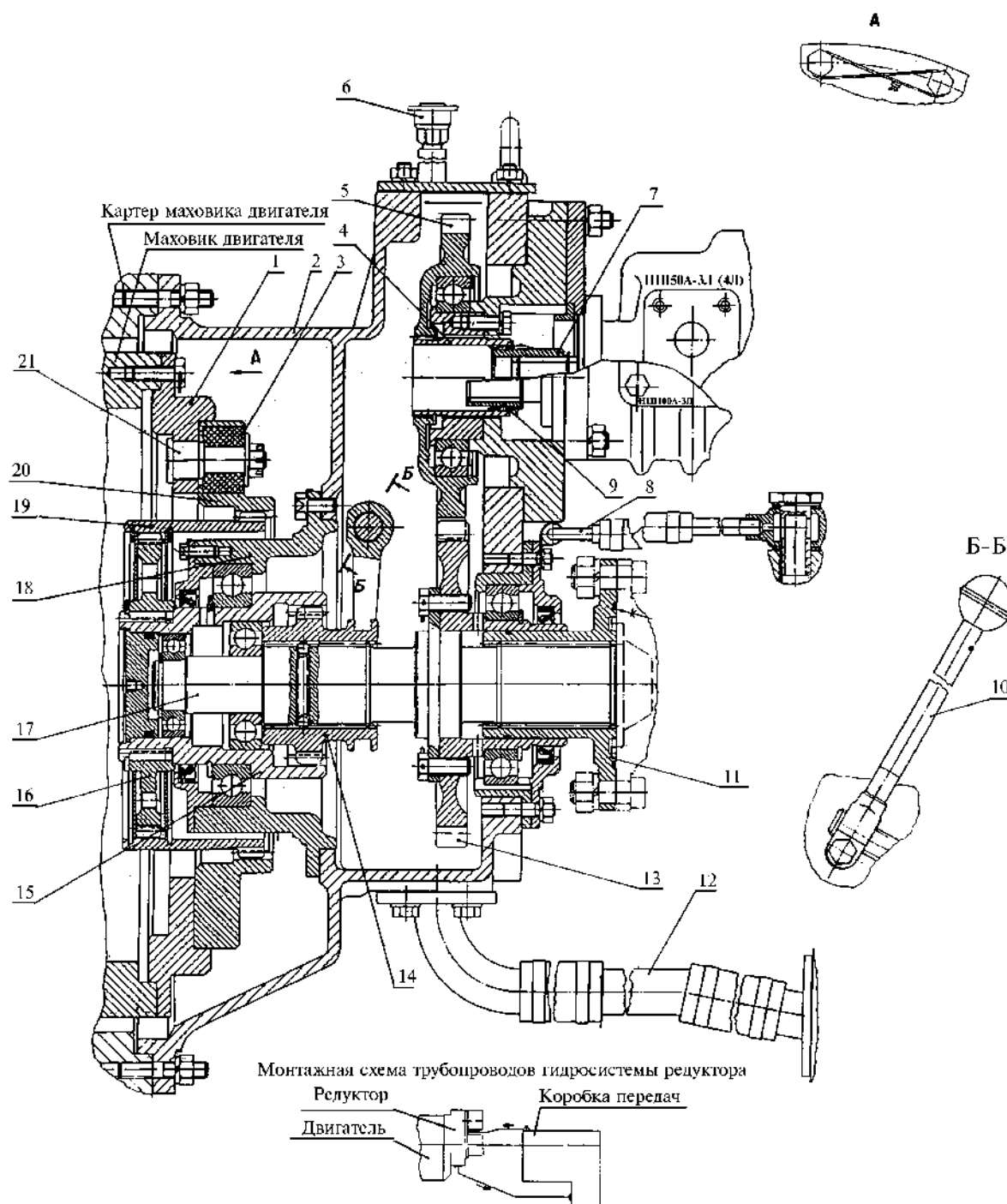
Рис. 25. Полужёсткая муфта и редуктор привода насосов
