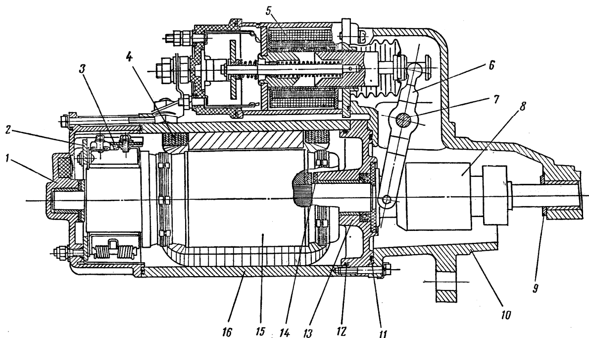
Рис. 62. Стартер
