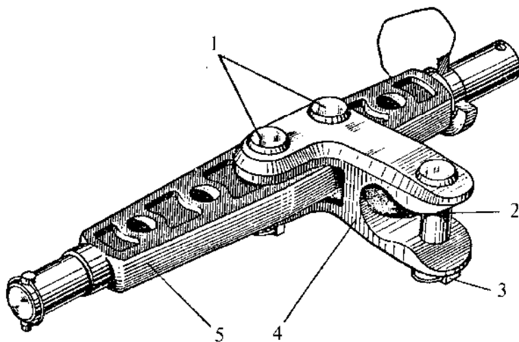
Рис. 60. Скоба прицепная
