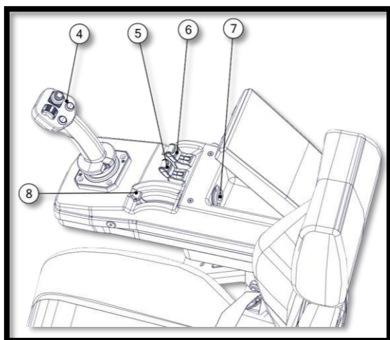
Рис. 89 – Правый модуль управления.
