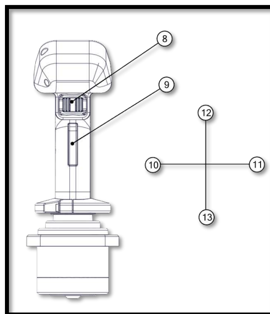
Рис. 87 Многофункциональный джойстик управления КП и гидравликой
