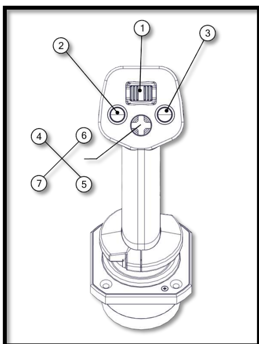
Рис. 86 Многофункциональный джойстик управления КП и гидравликой
