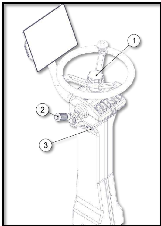
Рис. 81 – (1) Зажим регулировки рулевого колеса по высоте. (2) Подрулевой переключатель. (3) Кнопка фиксации угла наклона рулевой колонки.
